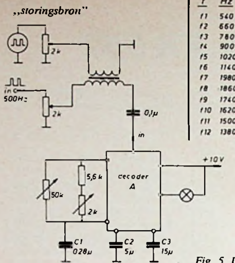
Fig. 5. Dubbeltoonopstelling.
